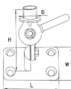
AISI316 BASE A DOPPIO SNODO
